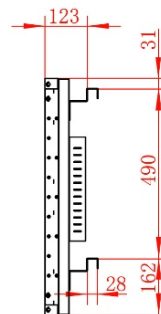
20X40 Hook
