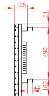
40X40 Hook
